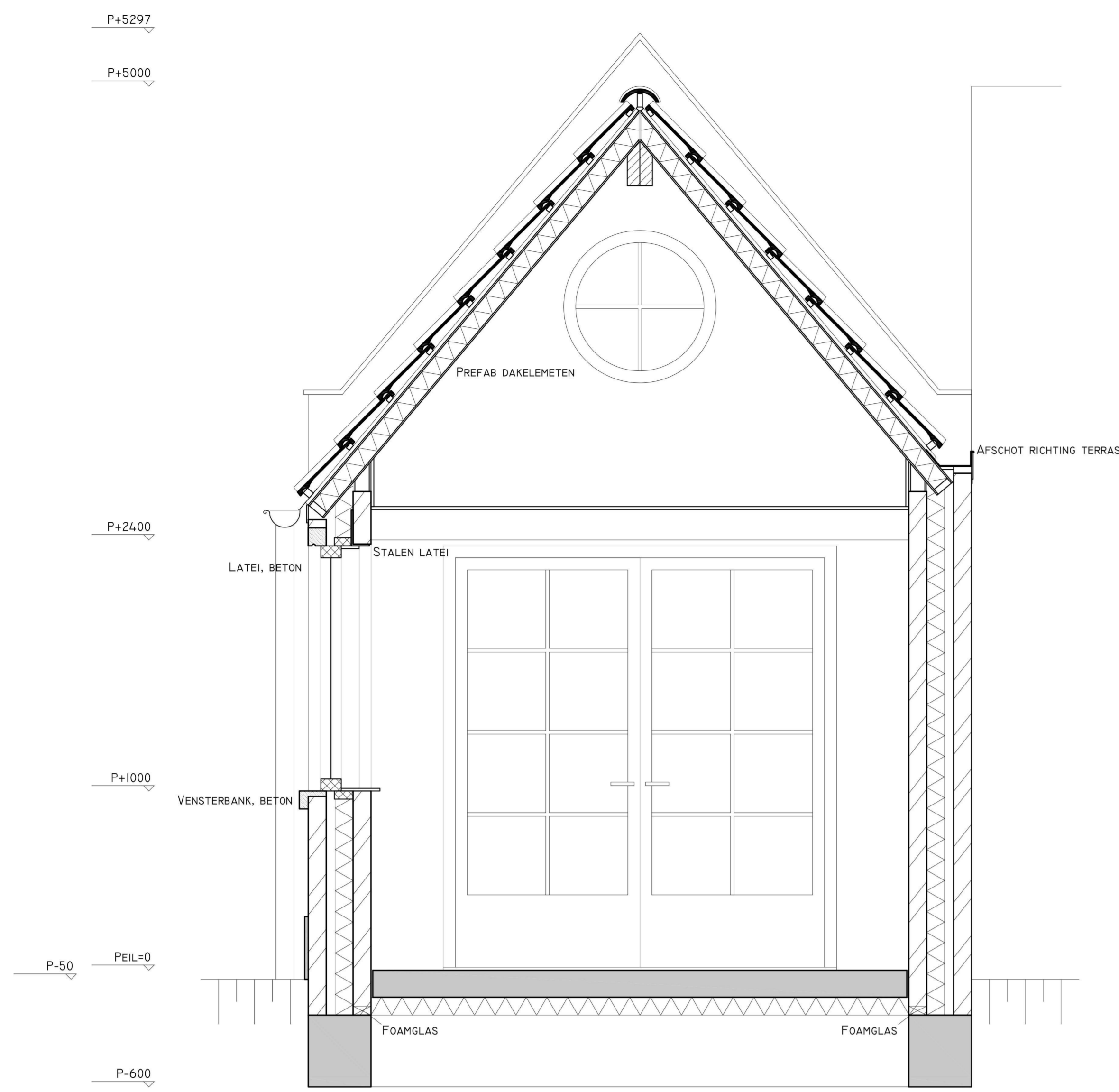
DOORSNEDE A-A'
