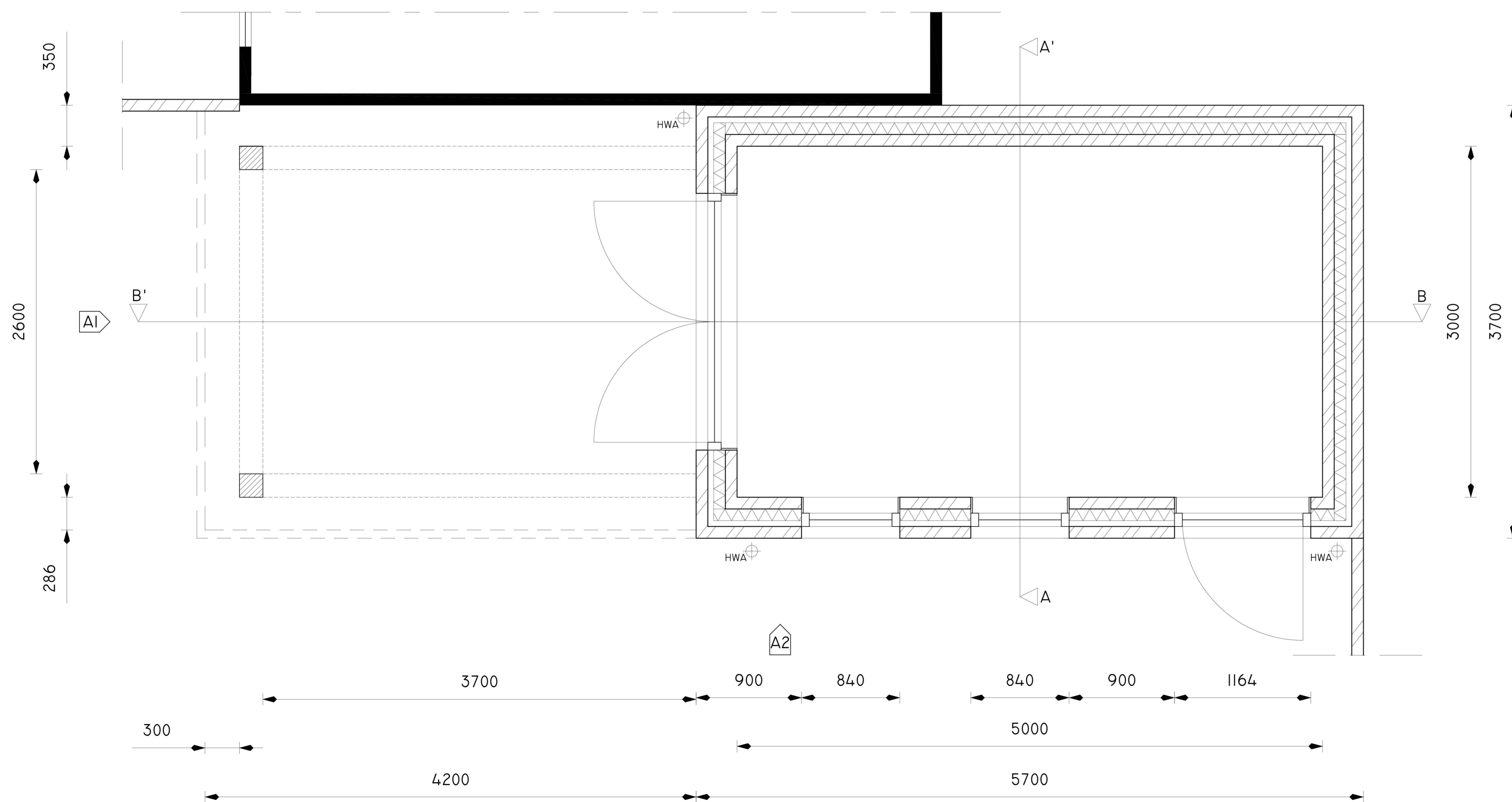
PLATTEGROND
