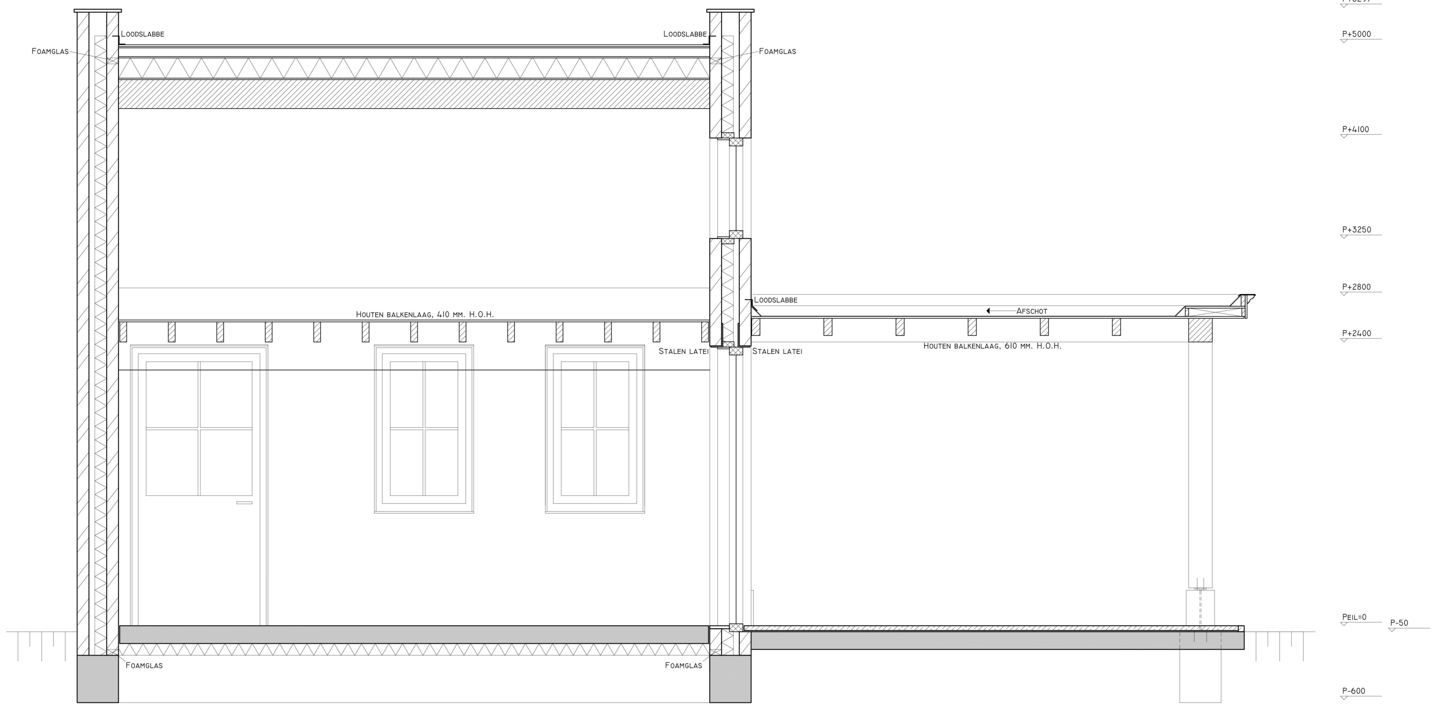
DOORSNEDE B-B'
